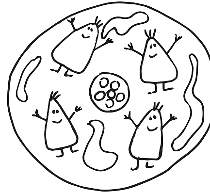
Enzyme in der Körper-Zelle
